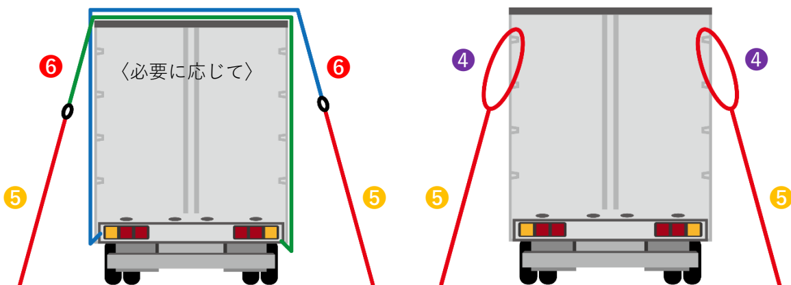
④ ナイロンロープ（20m/m） ⑥ オーバーラッシングベルト
